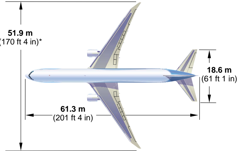
767-400ER
