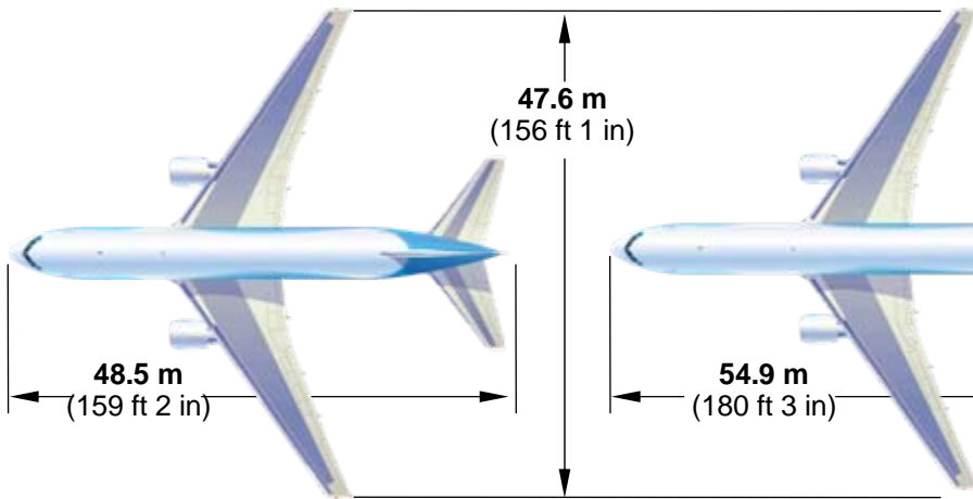
767-200ER
